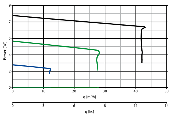
CURVE ASSORBIMENTI
