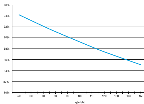
HRI-E ONE EFFICIENZA
