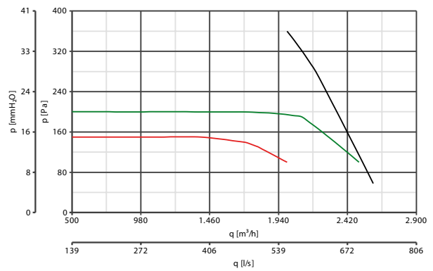
NRG HE 2000 cod. 45124 Funzionamento a portata costante
