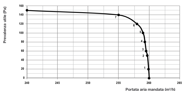
VORT HRI 260 DH VENTILATORE DI MANDATA
