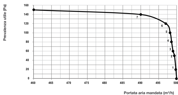
VORT HRI 500 DH VENTILATORE DI MANDATA
