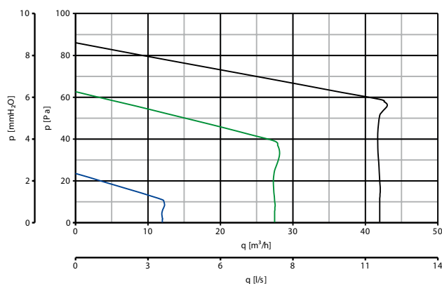
CURVE PORTATA/PRESSIONE
