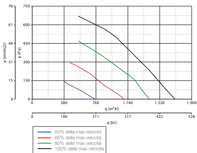
NRG HE 1000 cod. 45126 Funzionamento a pressione costante
