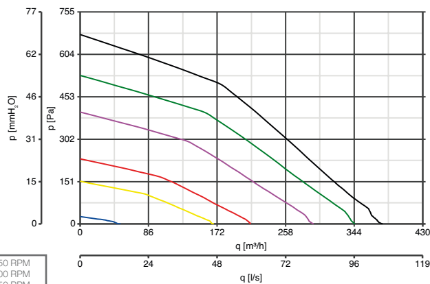
VORT PROMETEO PLUS HR 400 CURVE PORTATA/PRESSIONE
