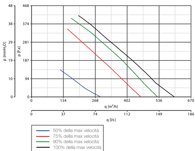
NRG HE 500 Cod. 45123 Funzionamento a pressione costante
